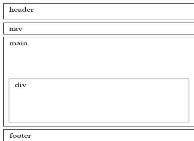
JavaJam wireframe
